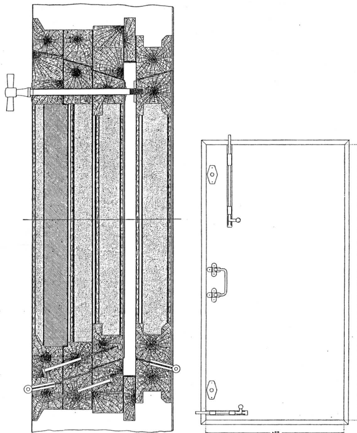
Abb. 13. Innere und äußere Tür der schalldichten Zelle (Horizontalschnitt \frac{1}{4} d. nat. Gr.). Reihenfolge der Schichten von oben. Innere Tür: 1. Wachstuch, 2. Wattin, 3. Blei, 4. Fournier, 5. Bast, 6. Ruberoid, 7. Asche, 8. Ruberoid, 9. Filz, 10. Bast, 11. Fournier, 12. Tuch. Äußere Tür: 1. Tuch, 2. Blei, 3. Fournier, 4. Ruberoid, 5. Asche, 6. Bast, 7. Fournier, 8. Ruberoid, 9. Bast, 10. Filz, 11. Ruberoid, 12. Asche, 13. Bast, 14. Ruberoid, 15. Fournier, 16. Bast, 17. Filz, 18. Ruberoid, 19. Kork, 20. Ruberoid, 21. Asche, 22. Bast, 23. Fournier, 24. Wachstuch.
